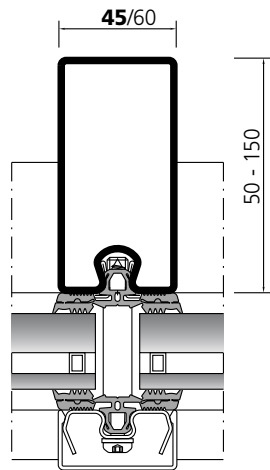
Vertikalfassade Brandschutz Façade verticale coupe-feu Fire-resistant curtain wall
