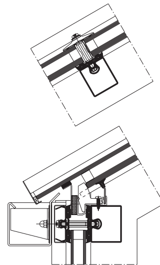
Schrägverglasung Verrière Sloped glazing
