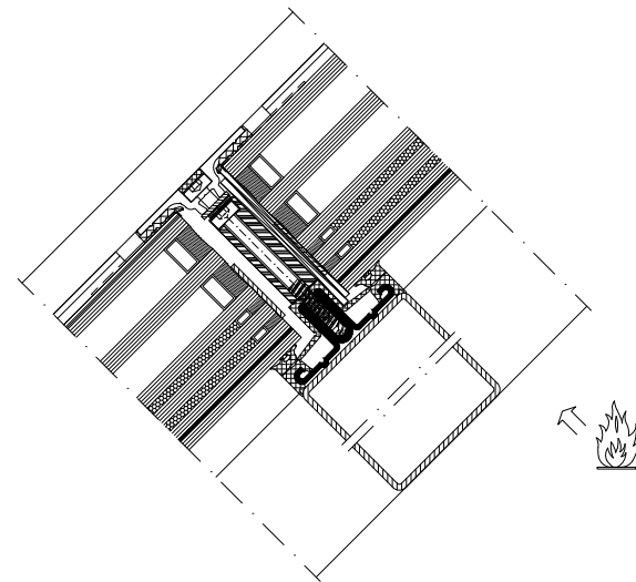
Schrägverglasung EI30/EI60 Verrière EI30/EI60 Sloped glazing EI30/EI60
