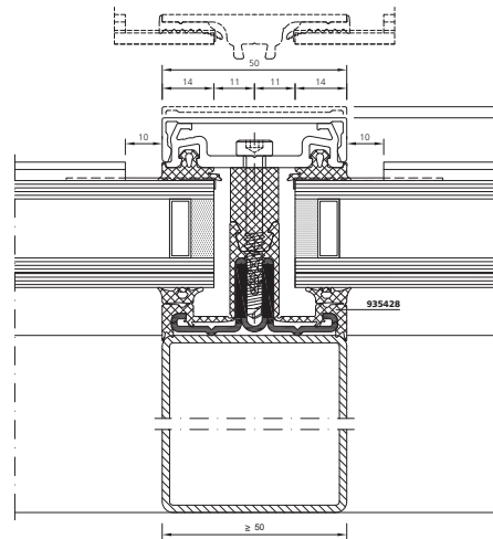
Schrägverglasung Verrière Sloped glazing
