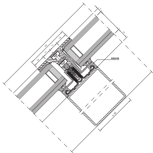
Schrägverglasung Verrière Sloped glazing
