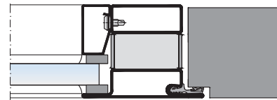
EI30 Tür mit Holztürblatt Porte EI30 avec vantail en bois Door EI30 with wooden door leaf
