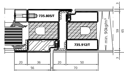
EI30 Durchschusshemmende Tür FB4 NS Porte coupe-feu et pare-balles EI30-FB4 NS Bulletproof fire resistant door EI30-FB4 NS
