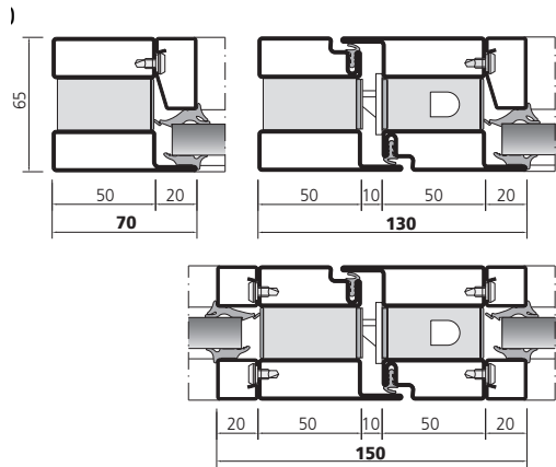
EI30 Tür Porte EI30 Door EI30
