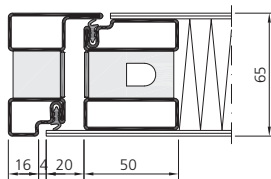
EI30 Blechtür Porte en tôle affleuré EI30 Flush mounted sheet metal door EI30
