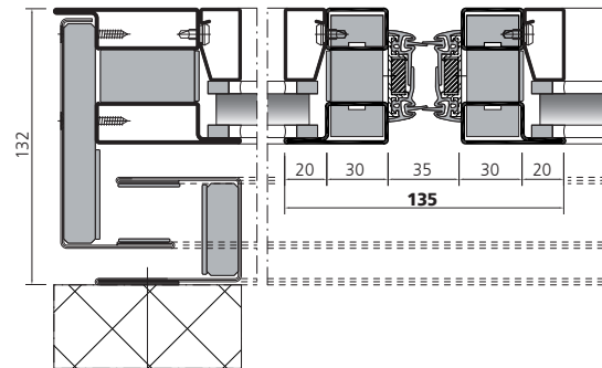
EI30 Schiebetür Porte coulissante EI30 Sliding door EI30
