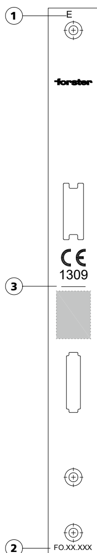
Tête de serrure à mortaiser
