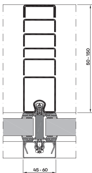
Transom
