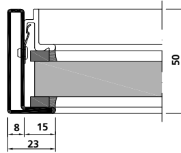
Festverglasung
