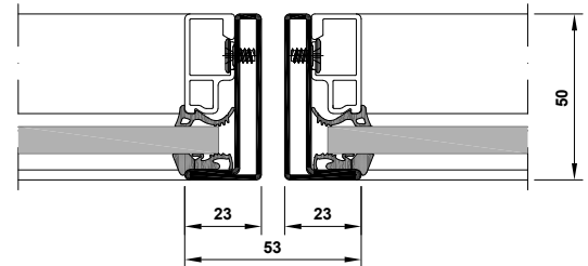
Übergang Festverglasung/Türflügel
