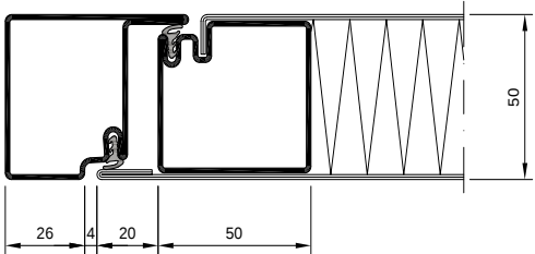
Vantail de porte et dormants combinés en tôle affleurée
