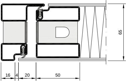
Vantail de porte et dormants combinés en tôle affleurée
