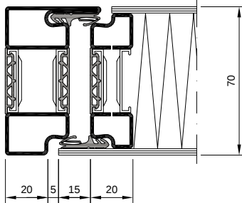
Vantail de porte et dormants combinés en tôle affleurée
