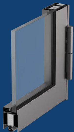
forster fuego light EI30/EI60 jusqu'à RC3
