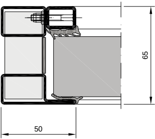
Vitrage fixe
