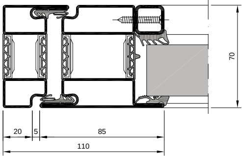
Türflügel Blendrahmenkombination verglast
