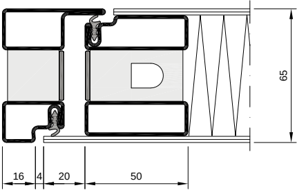
Türflügel Blendrahmenkombination flächenbündig verblecht
