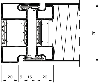
Türflügel Blendrahmenkombination flächenbündig verblecht
