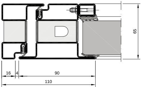
Türflügel Blendrahmenkombination verglast
